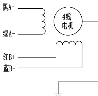
4线双极性电机
