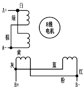
8线双极性·并联
