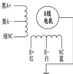
6线中线点连接
