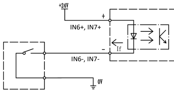
NPN 输入示意图
