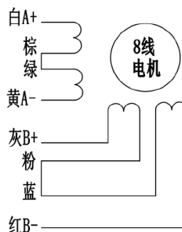
8线双极性·串联
