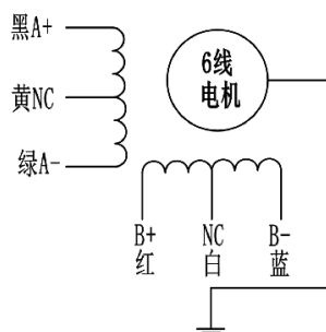
6线串行连接
