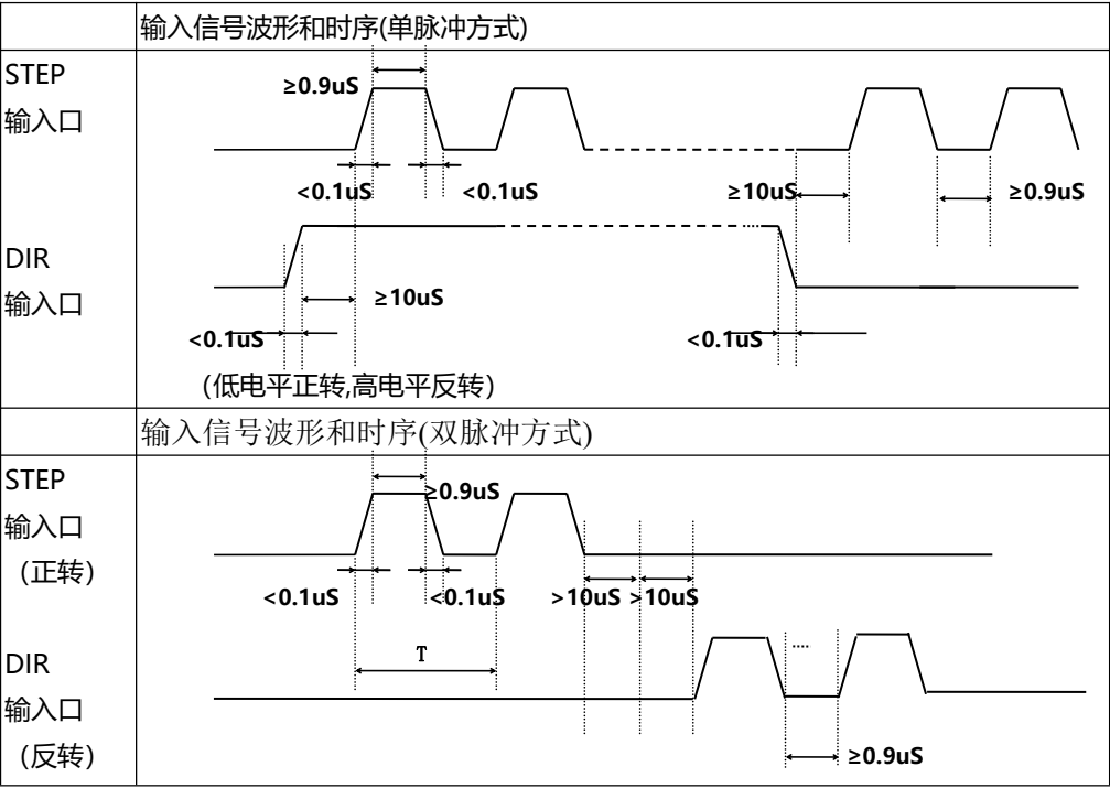
脉冲/方向输入时序图
